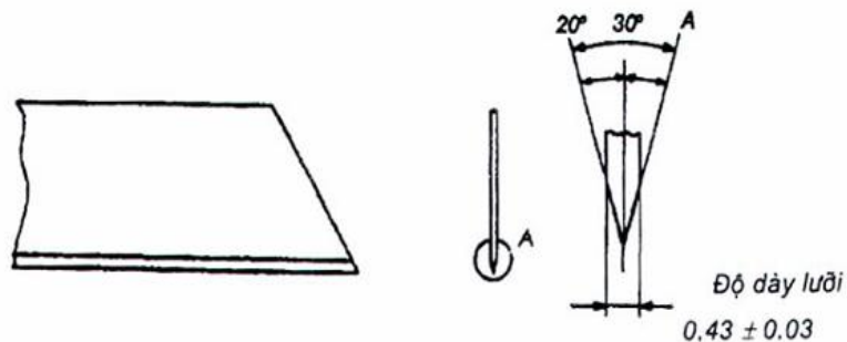
Hình 1 - Dao cắt
